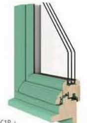
R30C1R + pièce d'appui
